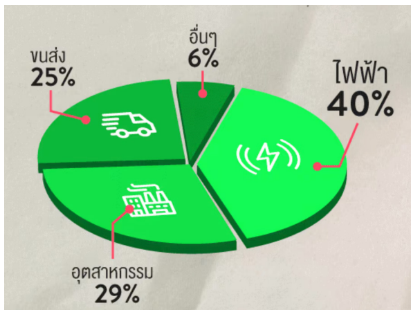
สัดส่วนการปล่อยก๊าซ \text{CO}_2 จากการใช้พลังงาน รายสาขาเศรษฐกิจ
