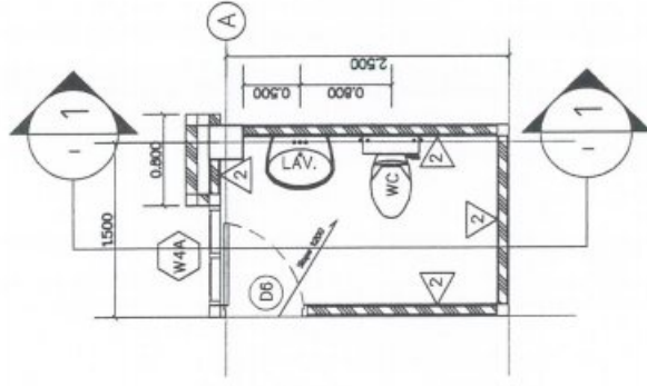
แบบขยายห้องน้ำห้องผู้ดูแลอาคาร
