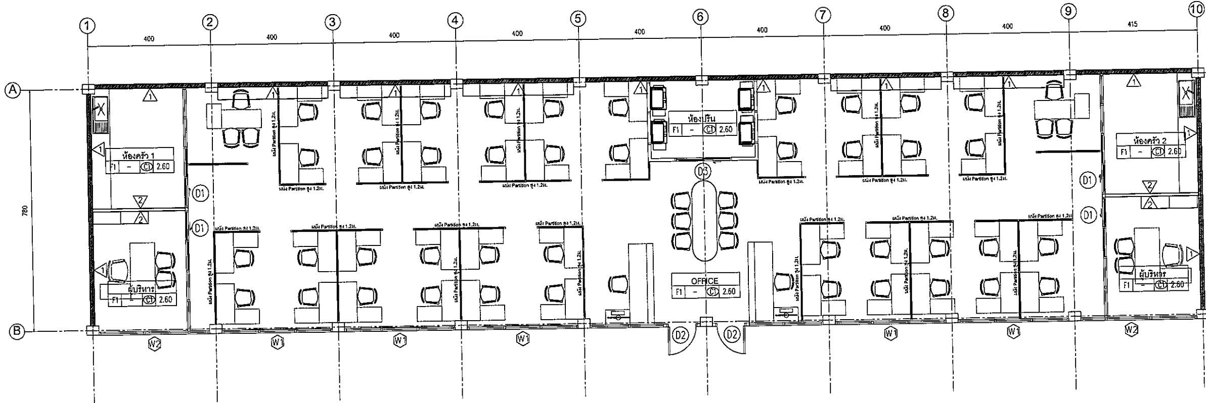
แปลนพื้นชั้น 2 มาตราส่วน 1:100 (แบบปรับปรุง อาคาร 2)
